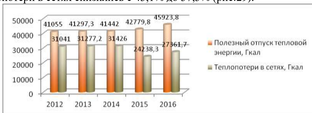
Рис.29. Показатели теплоснабжения
